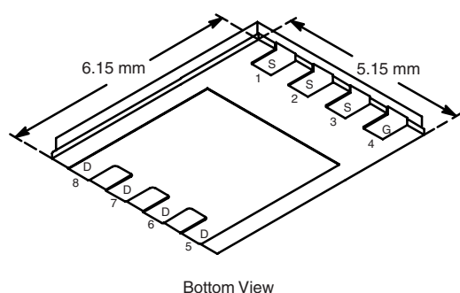
PowerPAK SO-8
