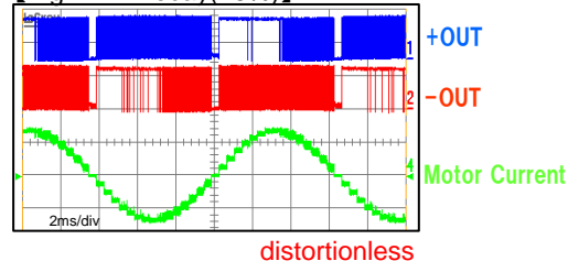
【Fig2:Mix Decay(25%)】
